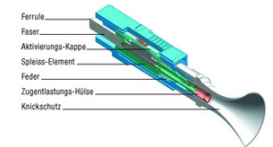
Abbildung 2.5: Stecker Aufbau
