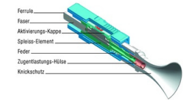
Abbildung 2.3: Stecker Aufbau
